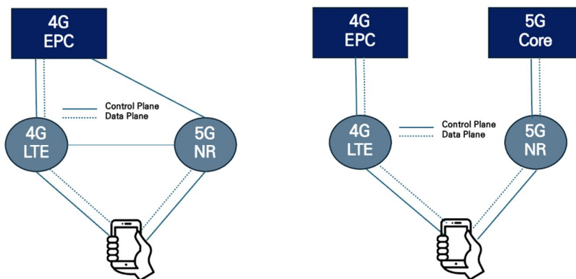
그림 3-2-1. 5G NSA vs 5G SA 구조 비교 다이어그램 (왼쪽: 5G NSA 오른쪽: 5G SA)
